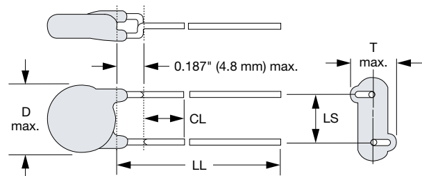
Fig. 2 - Inline wire
