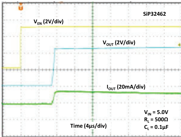
Fig. 33 - Turn-on Time
